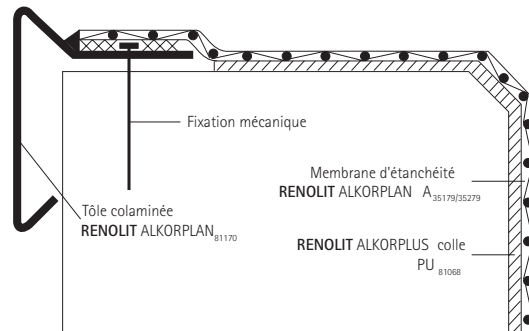
Fig.4: Collage en plein de la membrane RENOLIT ALKORPLAN A
