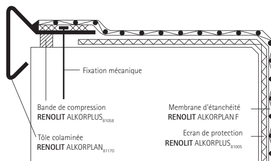
Fig. 5: Etanchéité au vent par pose en indépendance d'autres membranes RENOLIT ALKORPLAN.
