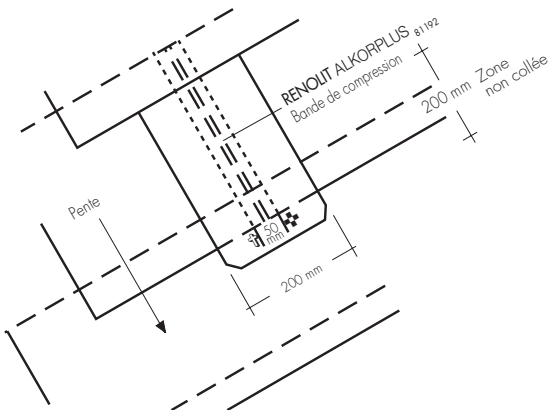
Fig.3: Jonction entre fins de rouleaux
